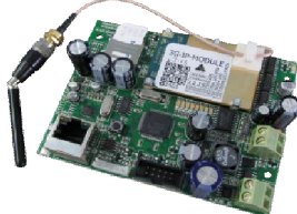
3G-IP-MODULE
